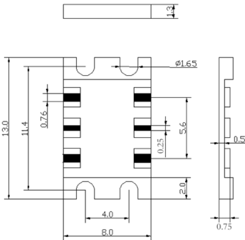
载片尺寸图（mm）：
