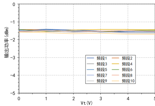
RF/N输出功率 VS Vt (N=16)
