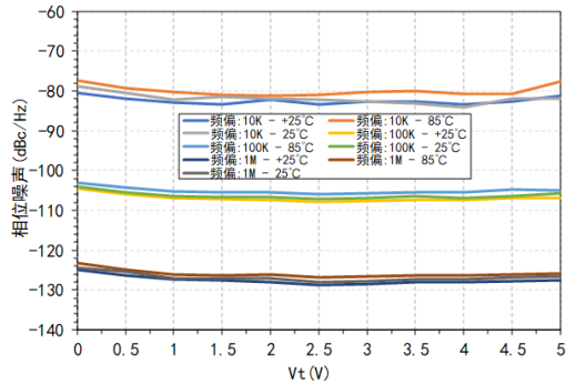
RFOUT相位噪声 VS Vt @频段10
