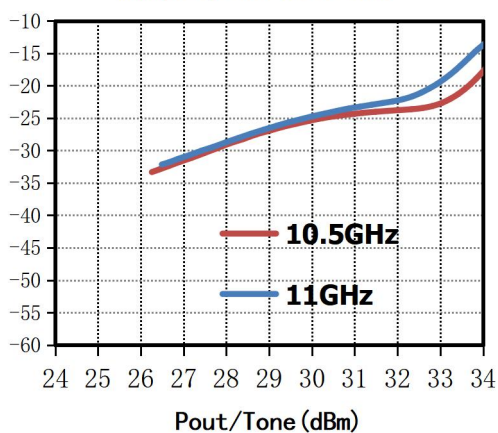
IM3 (dBc) vs. Pout/Tone
