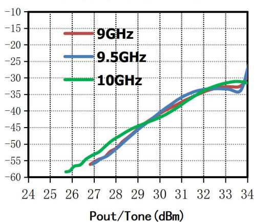
IM5 (dBc) vs. Pout/Tone
