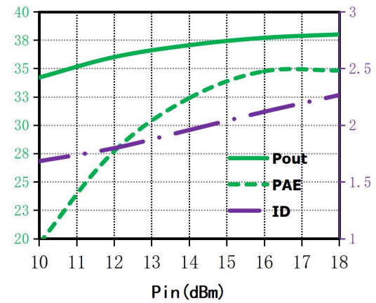
Pout (dBm) 、PAE (%)、ID(A) vs. Pin,f=9.5GHz
