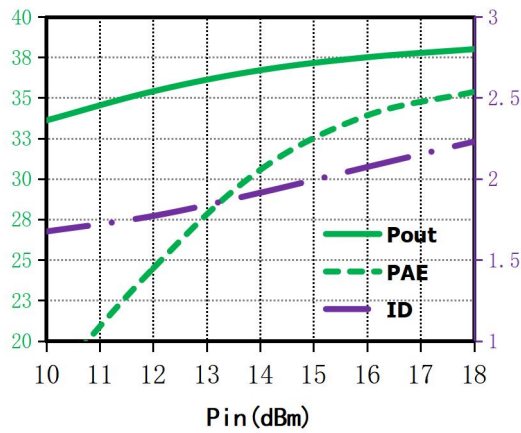
Pout (dBm) 、PAE (%)、ID(A) vs. Pin,f=9GHz
