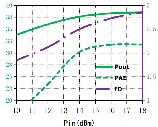
Pout (dBm) 、PAE (%)、ID(A) vs. Pin,f=10.5GHz
