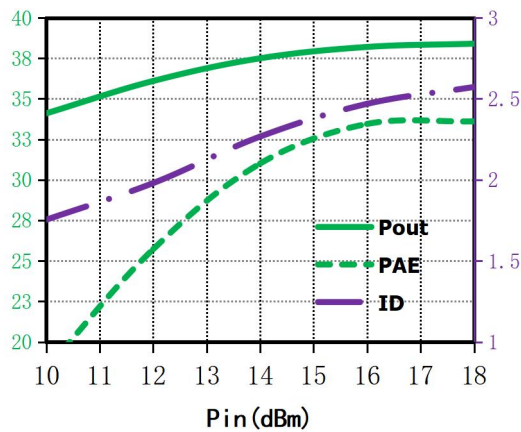
Pout (dBm) 、PAE (%)、ID(A) vs. Pin,f=10GHz
